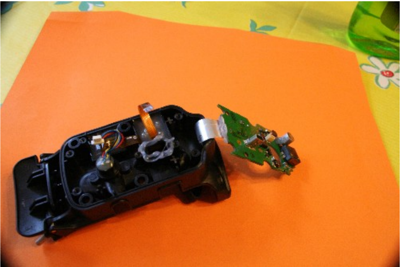
Silicon an USB-Anschluß und Flachbandstecker(von der Unterseite)
