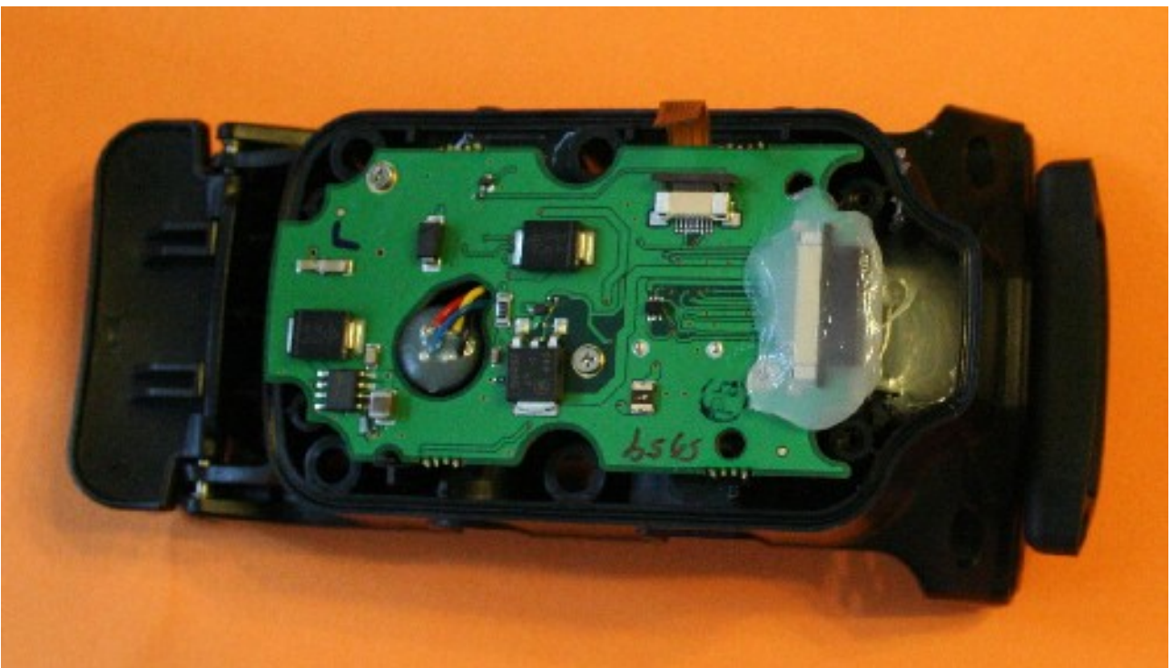
Silicon an Flachbandstecker und Zuleitung
